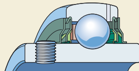
Innenring mit zwei Gewindestiften
